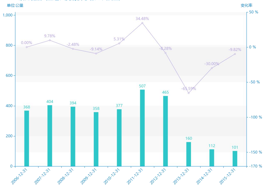
2006-2015液化石油气管道长度规模与增长率(公里)
