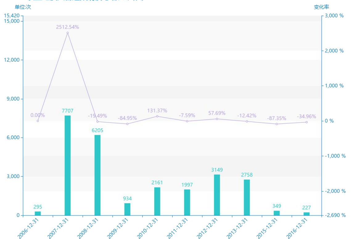
2006-2016发生地质灾害起数规模与增长率(次)
