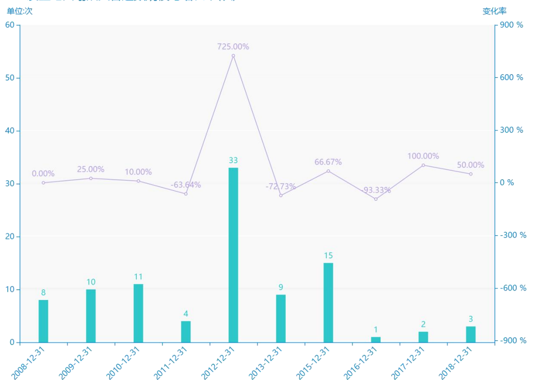
2008-2018发生地面塌陷灾害起数规模与增长率(次)
