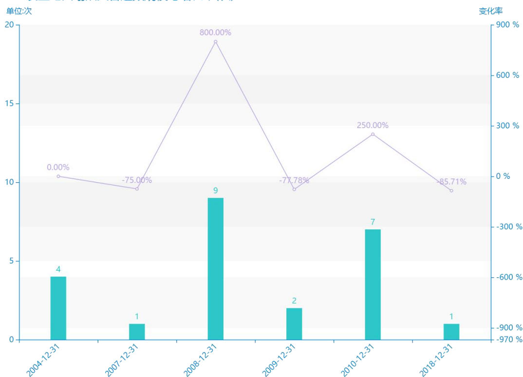
2004-2018发生地面塌陷灾害起数规模与增长率(次)
