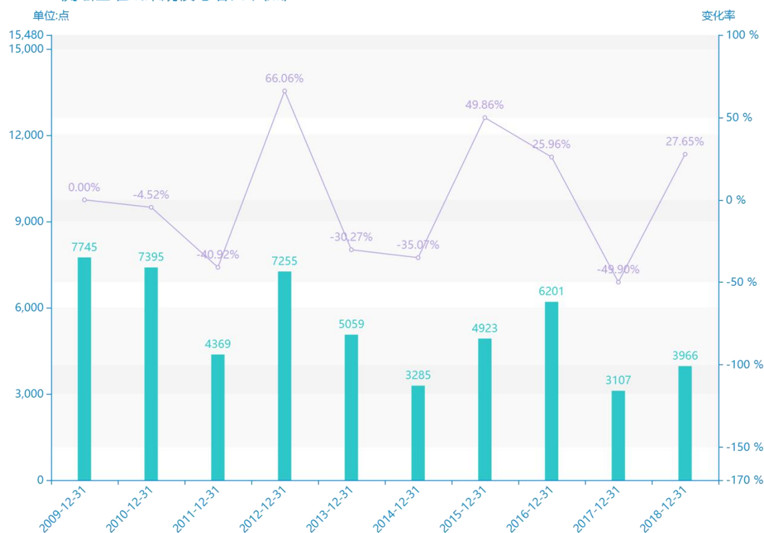
2009-2018测绘基准成果规模与增长率(点)
