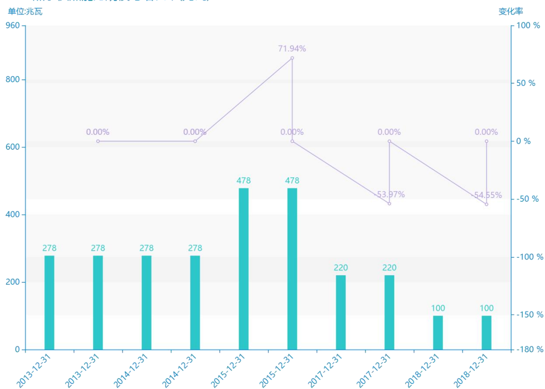
2013-2018热水供热能力规模与增长率(兆瓦)
