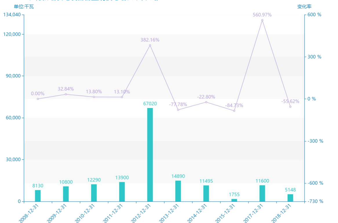
2008-2018农村新增发电设备容量规模与增长率(千瓦)
