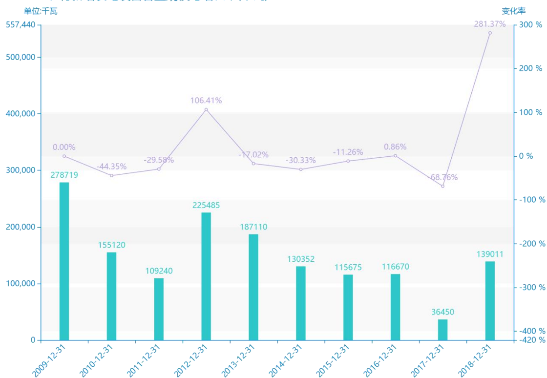
2009-2018农村新增发电设备容量规模与增长率(千瓦)
