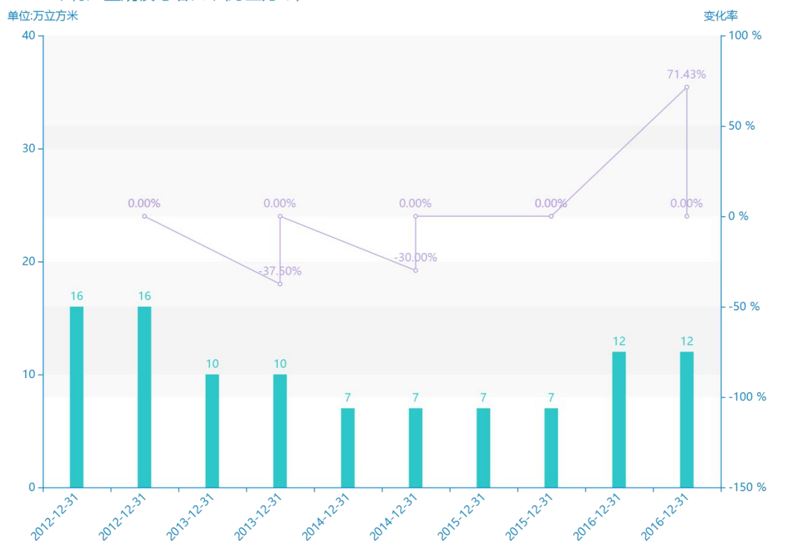
2012-2016木材产量规模与增长率(万立方米)
