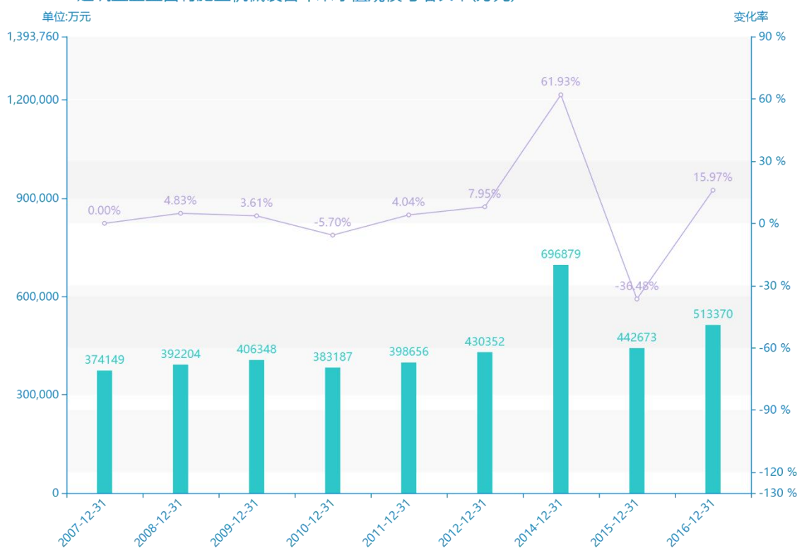
2007-2016建筑业企业自有施工机械设备年末净值规模与增长率(万元) 建筑业企业自有施工机械设备年末净值(万元) —○— 增长率
