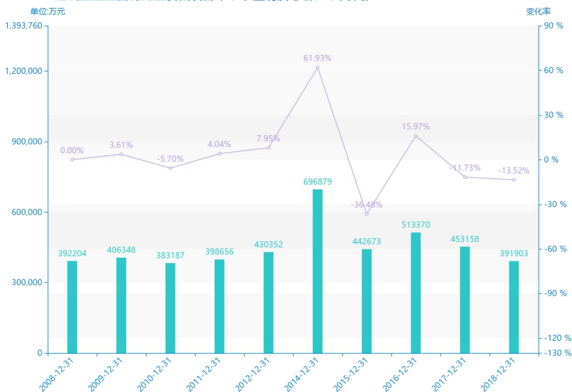
2008-2018建筑业企业自有施工机械设备年末净值规模与增长率(万元) ■ 建筑业企业自有施工机械设备年末净值(万元) —○— 增长率
