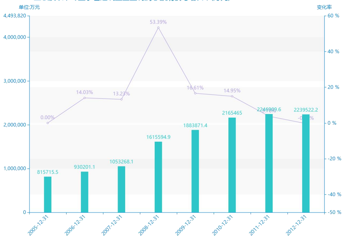
2005-2012三级及以下专业承包建筑业企业利润总额规模与增长率(万元) —○— 增长率
