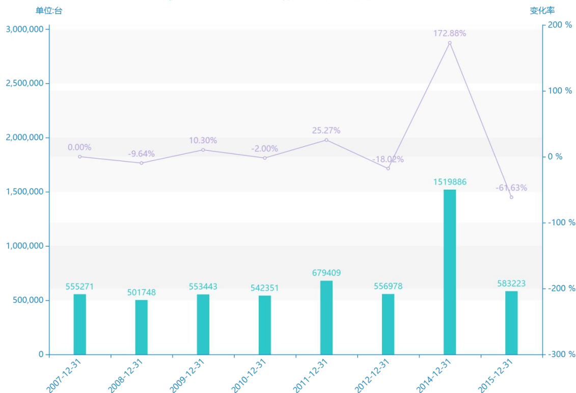
2007-2015建筑业企业自有施工机械设备年末总台数规模与增长率(台) 建筑业企业自有施工机械设备年末总台数(台) —○— 增长率
