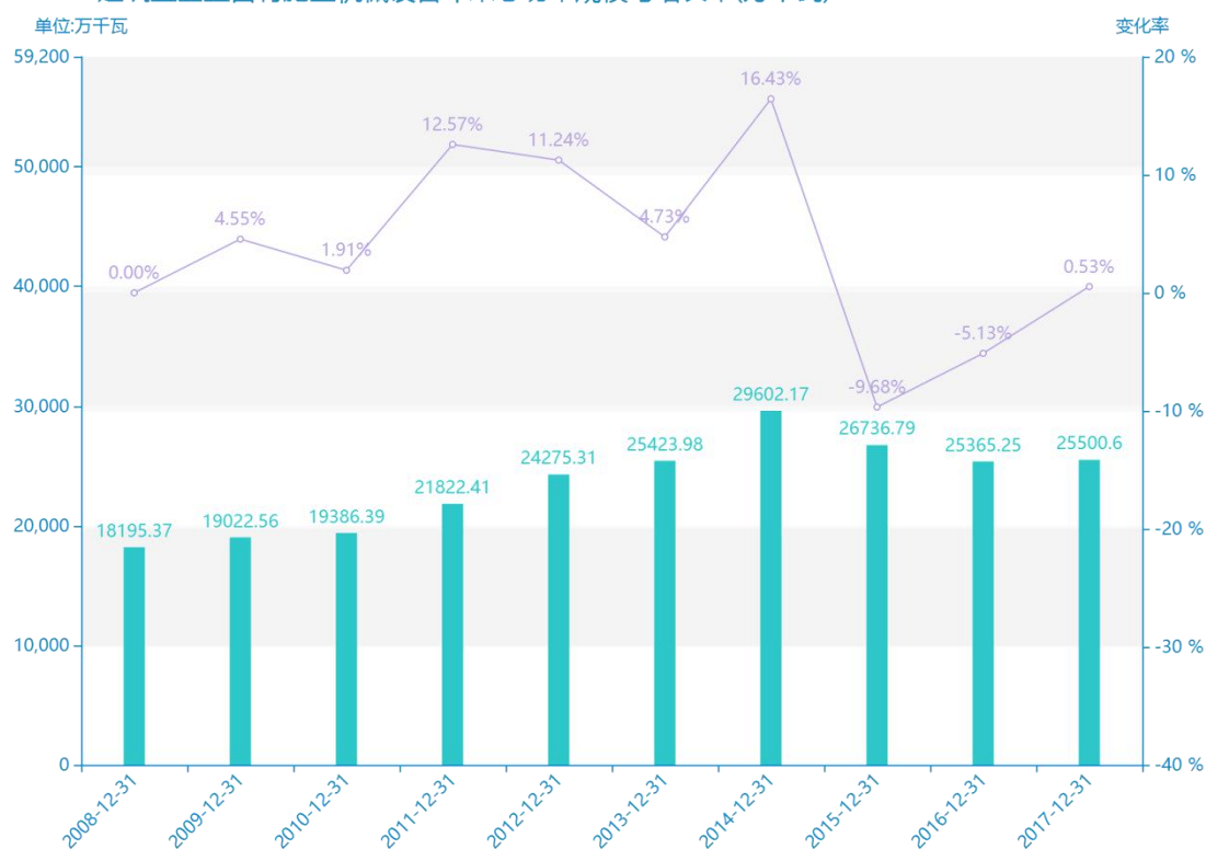
2008-2017建筑业企业自有施工机械设备年末总功率规模与增长率(万千瓦) — 增长率
