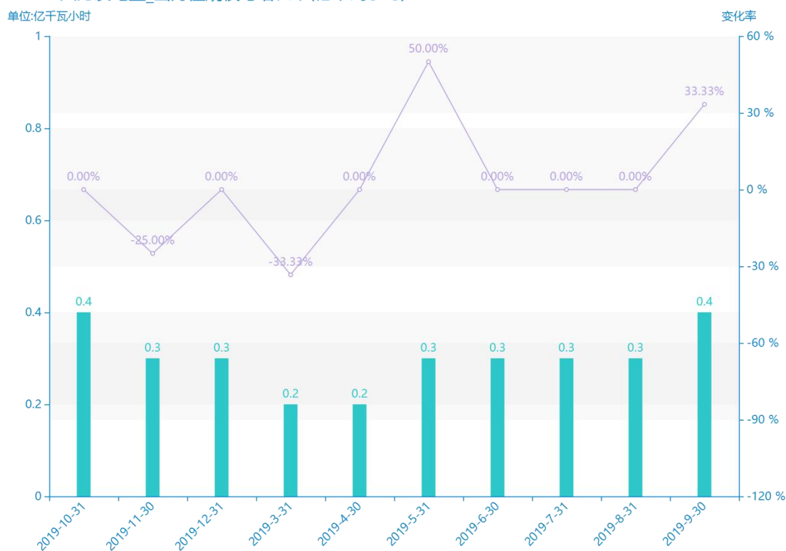
2019-2019火力发电量_当月值规模与增长率(亿千瓦小时)
