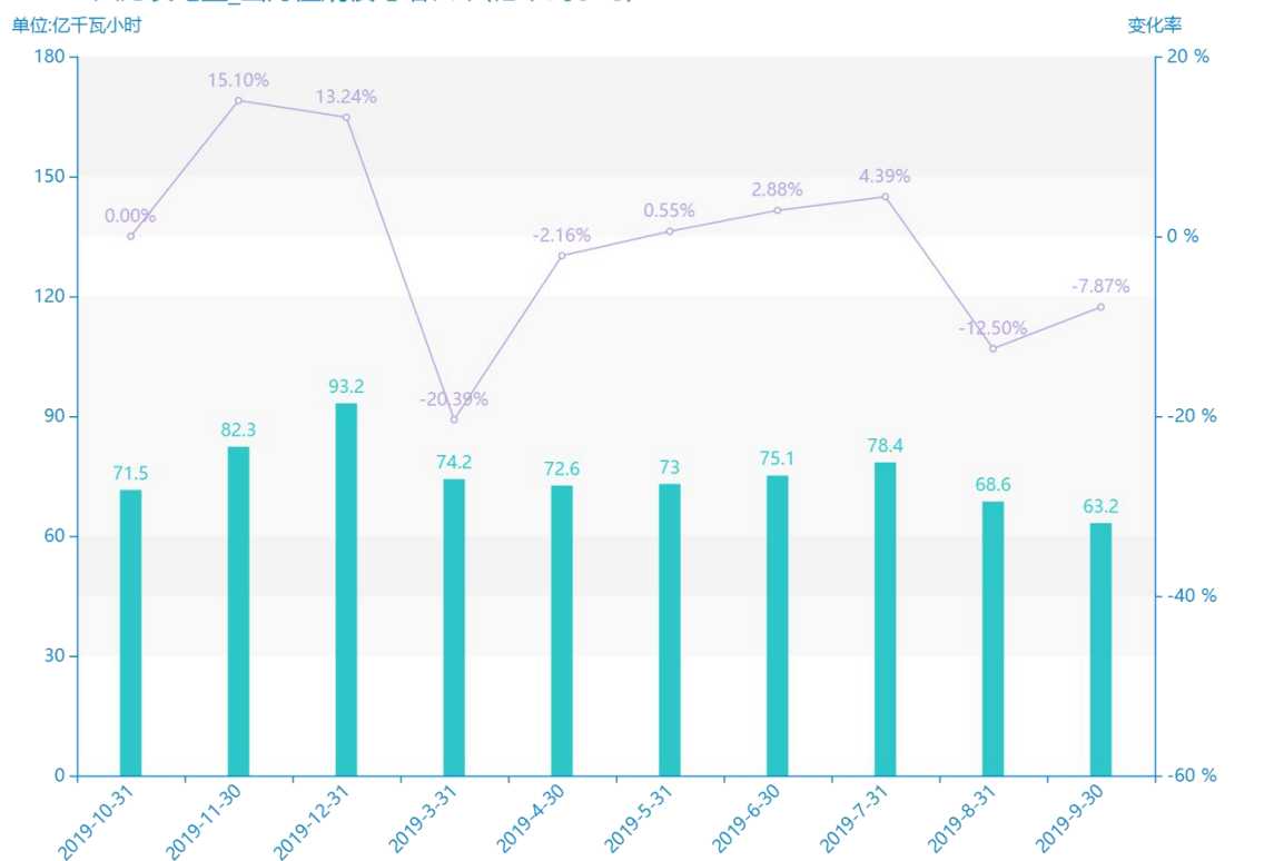
2019-2019火力发电量_当月值规模与增长率(亿千瓦时)
