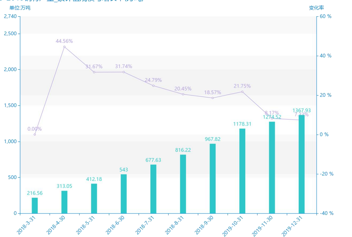
2018-2019钢材产量_累计值规模与增长率(万吨)
