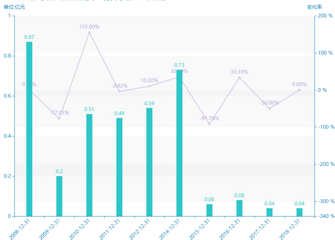
2008-2018外商独资建筑业企业资产规模与增长率(亿元)
