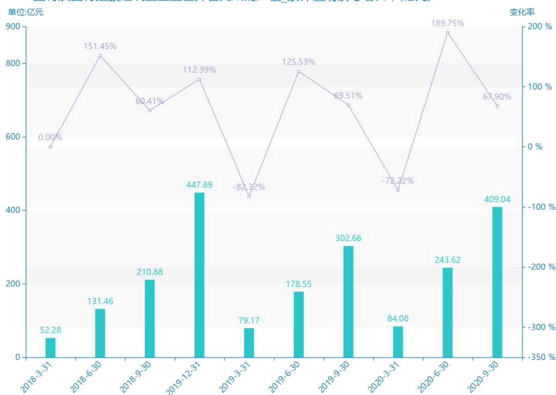
2018-2020国有及国有控股建筑业企业在外省完成的产值_累计规模与增长率(亿元)
