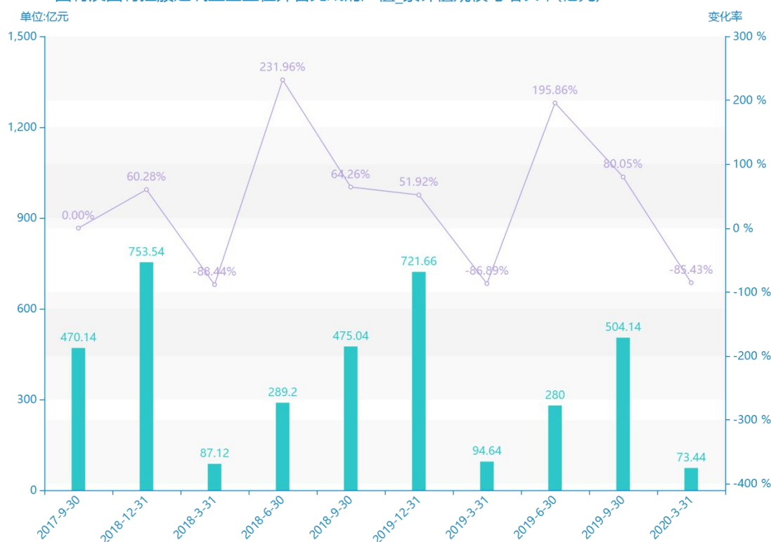
2017-2020国有及国有控股建筑业企业在外省完成的产值_累计规模与增长率(亿元)
