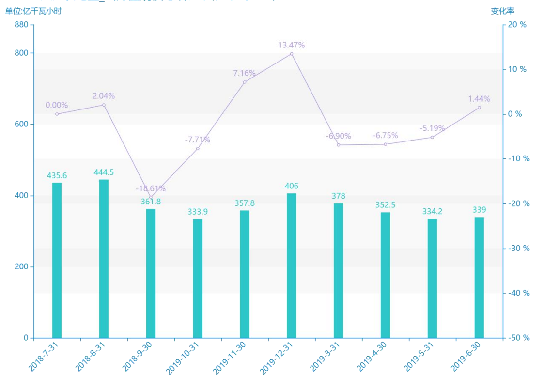
2018-2019火力发电量_当月值规模与增长率(亿千瓦小时)
