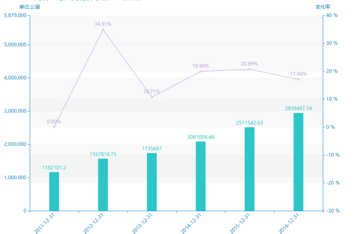
2011-2016光缆线路长度规模与增长率(公里)
