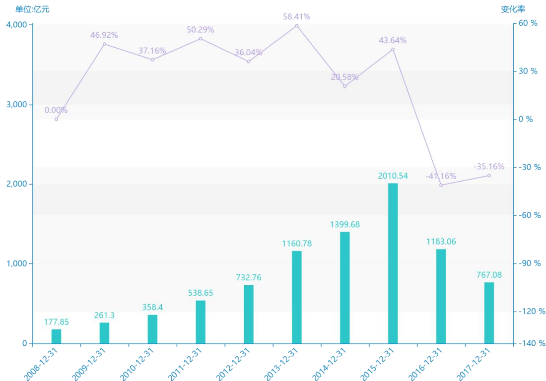
2008-2017电力、蒸汽、热水生产和供应业投资规模与增长率(亿元) ■ 电力、蒸汽、热水生产和供应业投资(亿元) —○— 增长率
